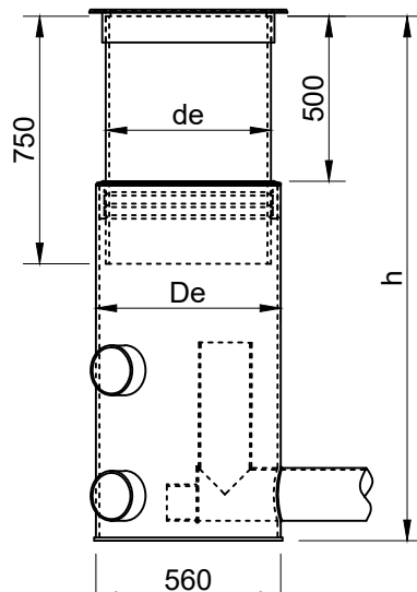
VIRTAUKSENSÄÄTÖKAIVO
